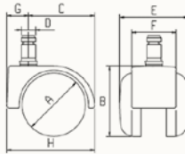
RADP+GPB Rueda Ø50 desmopan autofrenada con peso
